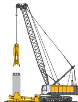
Pfahlbohrgreifer und Verrohrungsmaschine
